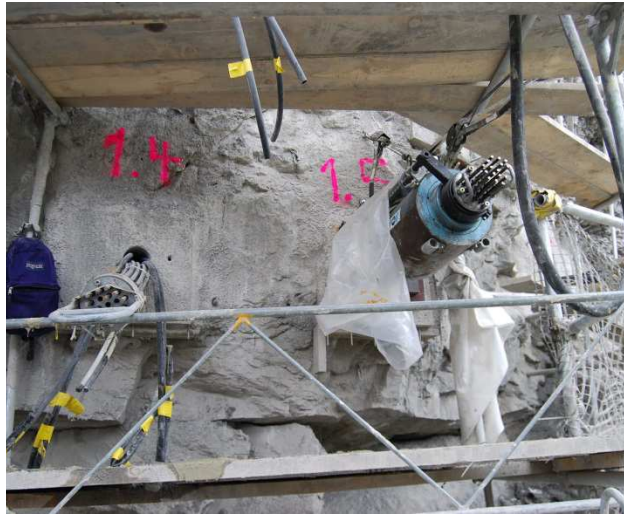
Einer von 10 Anker (Spannkraft ca. 250 to) zur Sicherung des Felsvorsprungs über dem Vortunnel.
